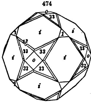
Achmatovak.
